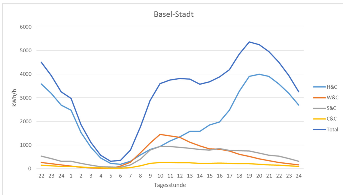
Abbildung 35: Leistungsprofil für den Kanton Basel-Stadt im Jahr 2030, COM Szenario
