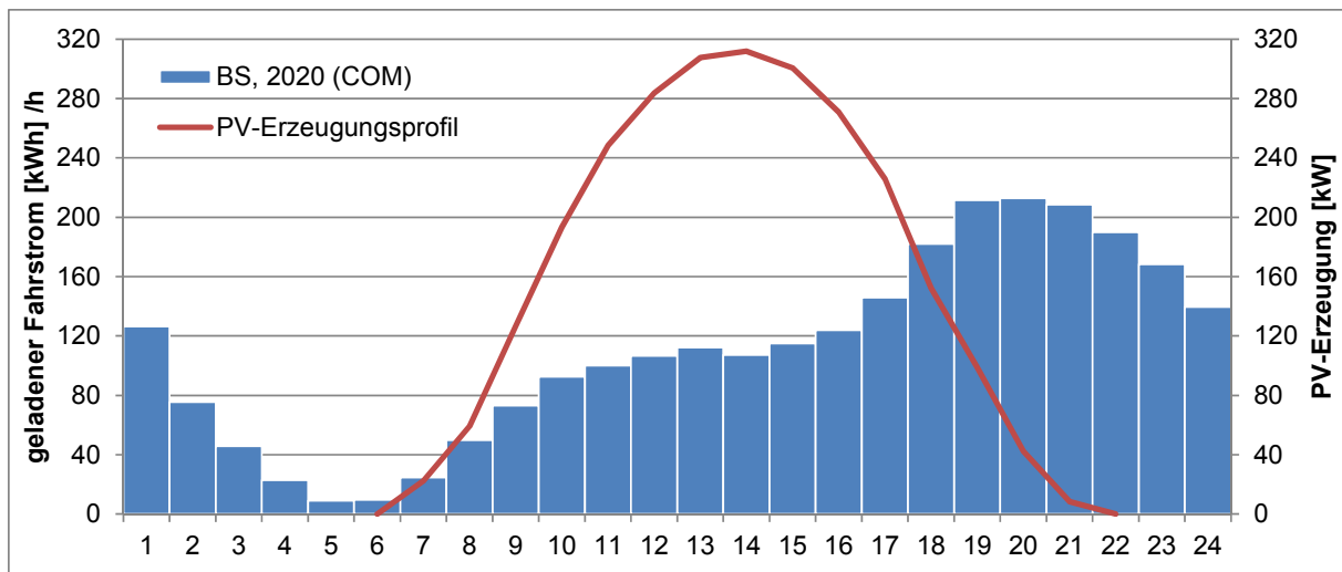
Abbildung 40: Gegenüberstellung des Tagesgangs von geladenem Fahrstrom für H&C und W&C mit einem prototypischen Photovoltaik-Erzeugungsprofil (PV-Erzeugung in der Abbildung entspricht der Menge des geladenen Stroms).
