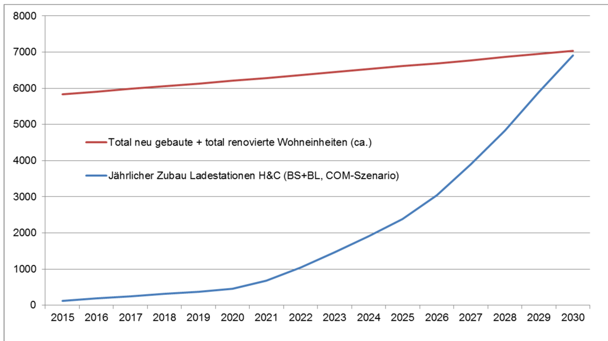
Abbildung 41: Gegenüberstellung der Anzahl jährlich neu zu erstellenden Anzahl H&C-Ladestationen und der geschätzten Anzahl jährlich neu gebauten oder total renovierten (1% des Gesamtbestandes) Wohneinheiten.
