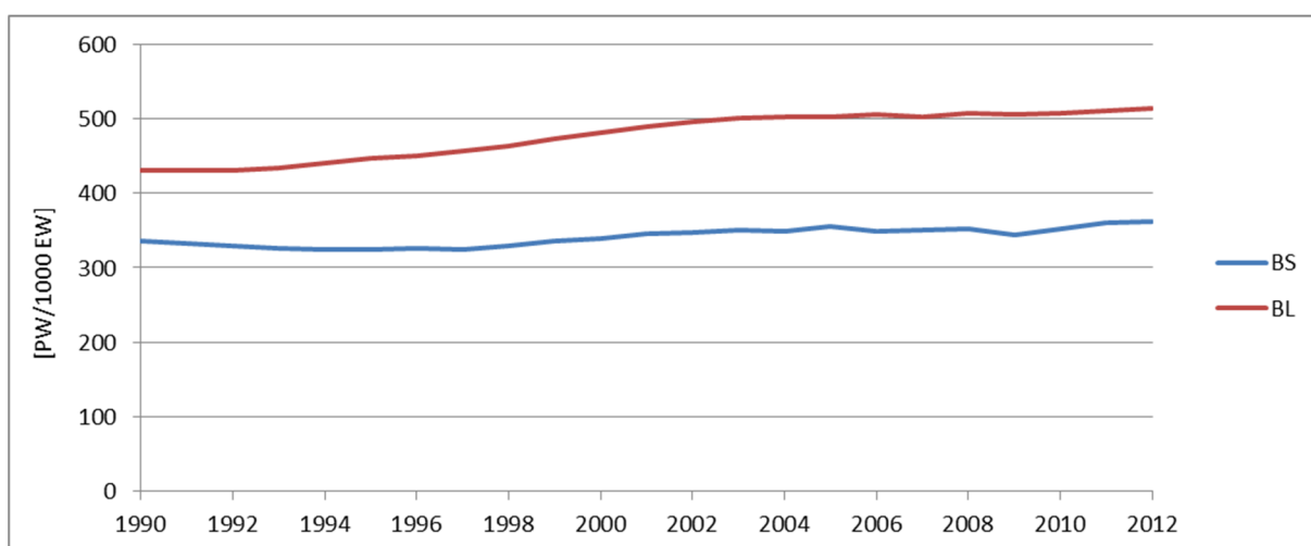
Abbildung 12: Historische Entwicklung des Motorisierungsgrades.
