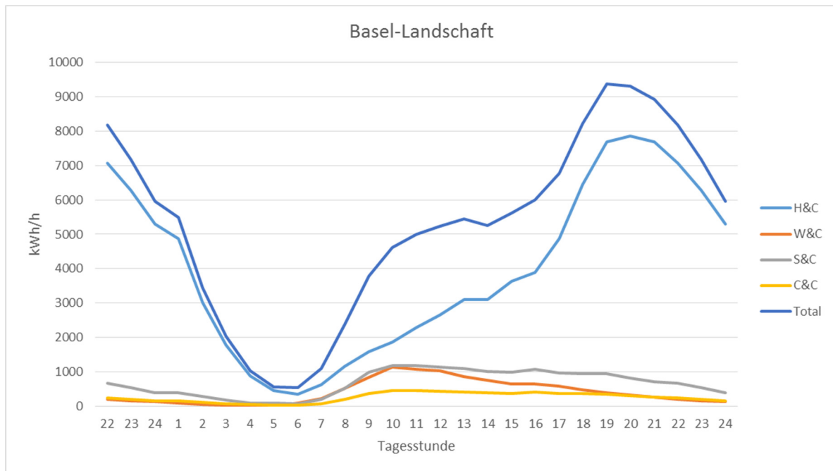
Abbildung 38: Leistungsprofil für Basel-Landschaft im Jahr 2030, COM Szenario
