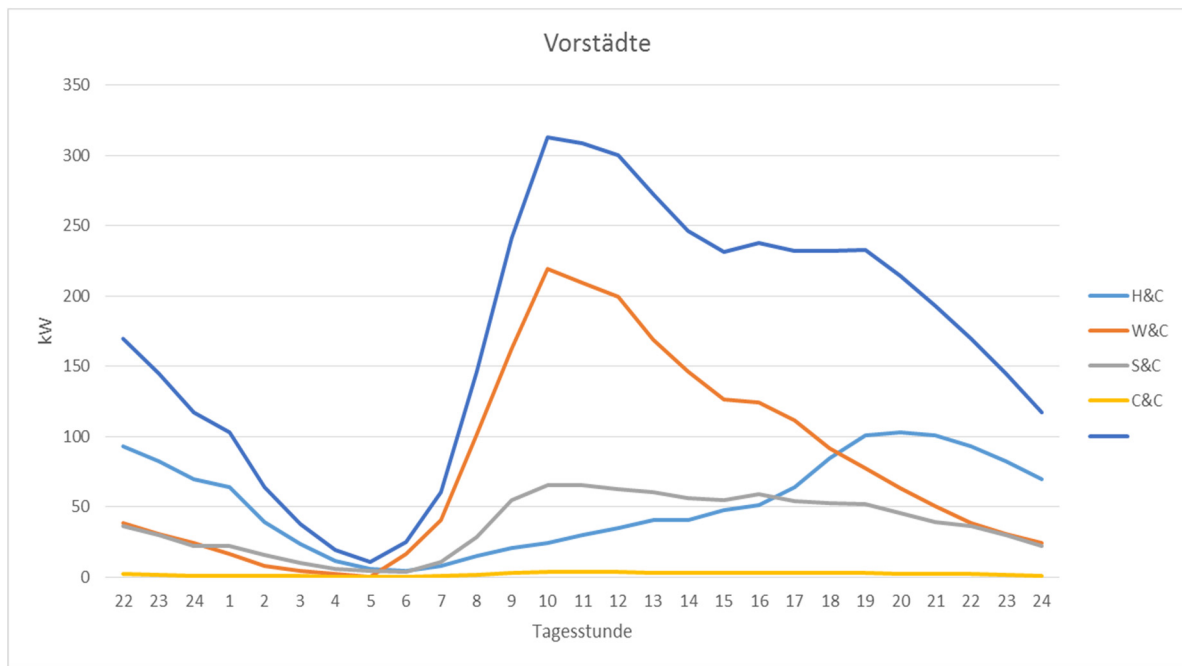
Abbildung 36: Leistungsprofil für Basel-Vorstädte im Jahr 2030, COM Szenario
