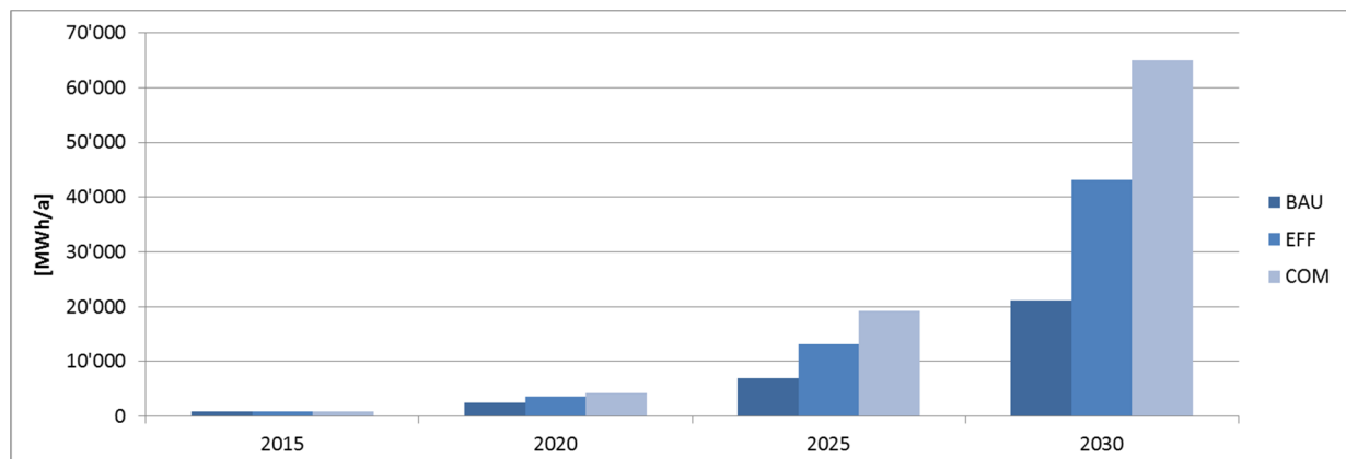
Abbildung 24: Verfahrere Strommenge in BS/BL je Jahr und Szenario.
