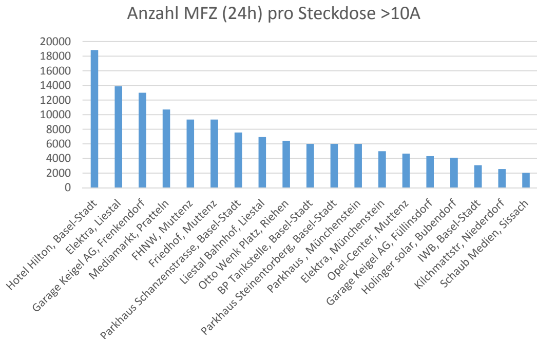
Abbildung 18: Geschätzte Verkehrsbelastung je Steckdose in unmittelbarer Nähe der bestehenden, öffentlichen Ladestationen in der Region Basel. Die Zahlen entsprechen dem durchschnittlichen Werktagsverkehr (DWV) heruntergebrochen auf eine Steckdose.
