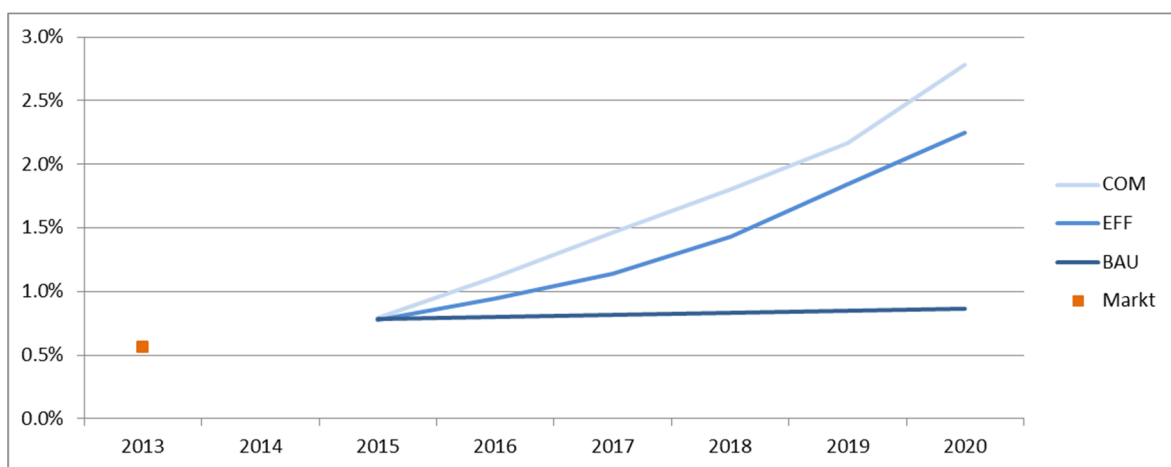
Abbildung 7: Marktanteil Elektrofahrzeuge 2013 vs. TA-SWISS Szenarien 2015-2020.
