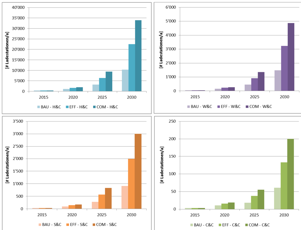
Abbildung 26: Anzahl Ladestationen je nach Ladestationstyp, Stichjahr und Szenario.
