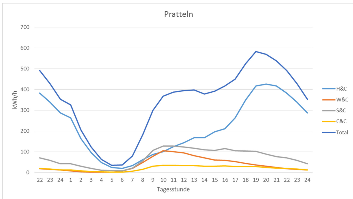
Abbildung 39: Leistungsprofil für Pratteln im Jahr 2030, COM Szenario
