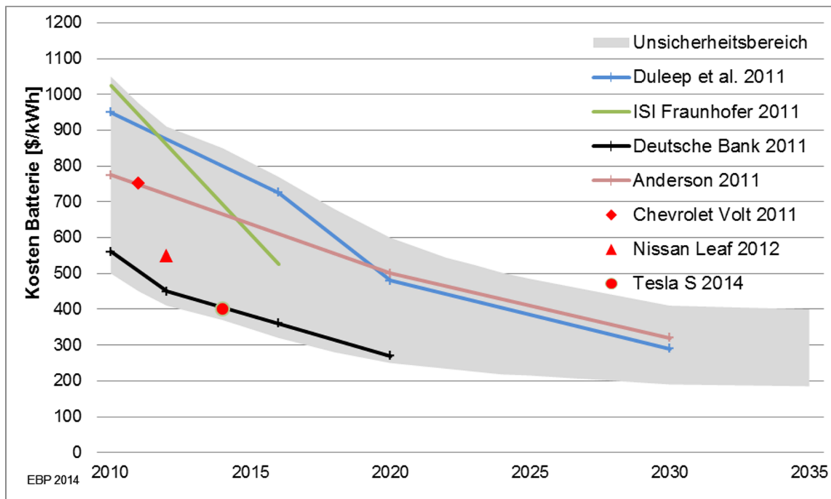
Abbildung 4: Aktuelle und prognostizierte Entwicklung der Kosten von Li-Ion-Batterien für Elektrofahrzeuge. Die Batteriekosten ausgewählter neuer Modelle sind einzeln dargestellt.
