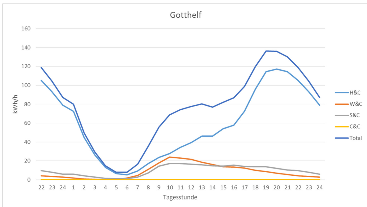
Abbildung 37: Leistungsprofil für Gotthelf im Jahr 2030, COM Szenario
