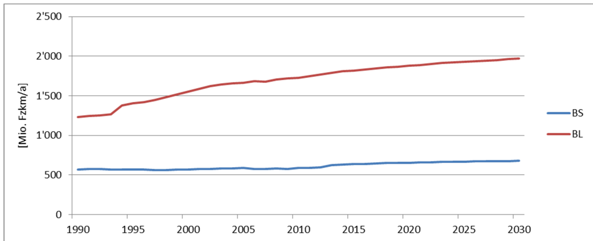
Abbildung 13: Jährliche Fahrleistungen (inklusive aussenkantonalen Verkehr) bis 2030.
