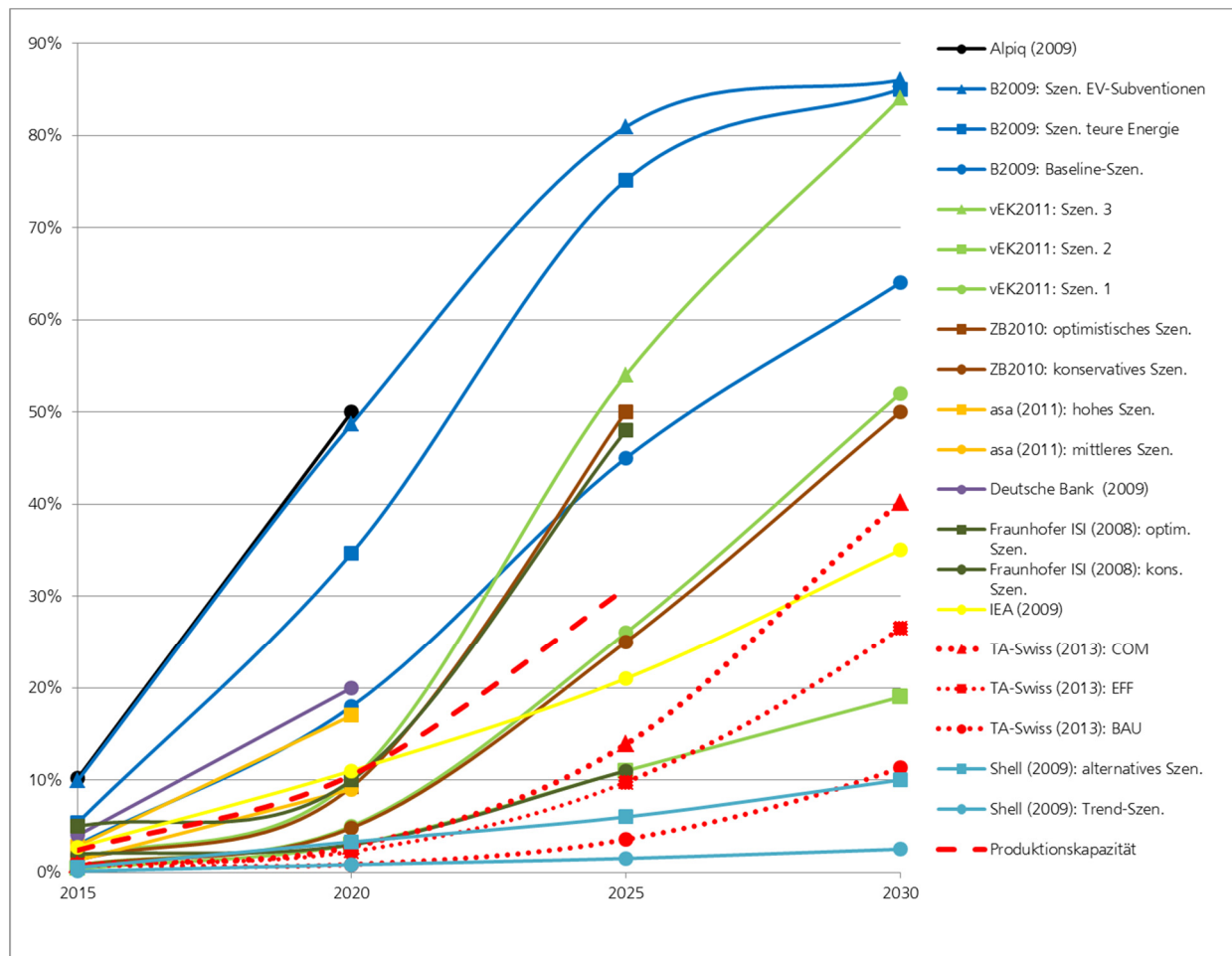
Abbildung 5: Spannweite der Marktpenetrationsszenarien für Elektrofahrzeuge aus der Literatur (inkl. weltweiter maximaler Produktionskapazität gemäss TA-SWISS [2013], rot gestrichelt).
