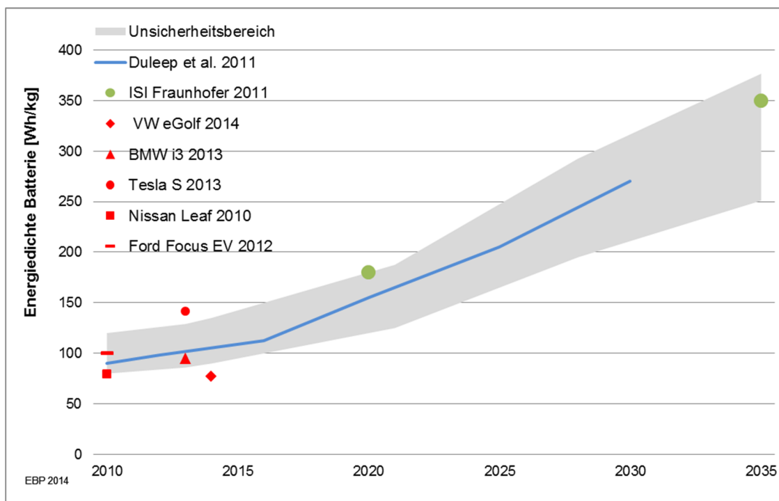
Abbildung 3: Aktuelle und prognostizierte Entwicklung der Energiedichte von Li-Ion-Batterien für Elektrofahrzeuge. Die Energiedichten ausgewählter neuer Modelle sind einzeln dargestellt.
