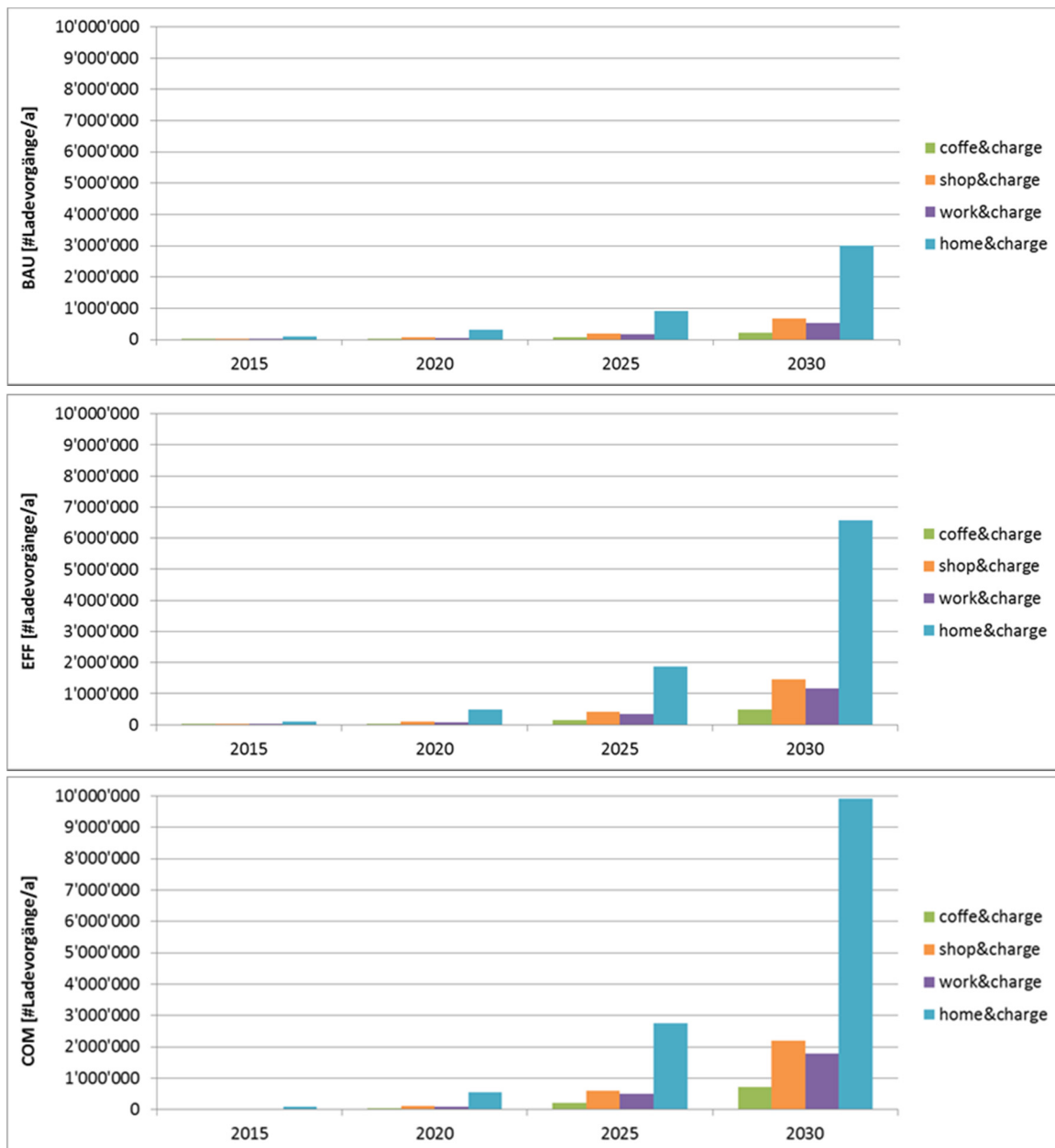
Abbildung 25: Anzahl Ladevorgänge je nach Szenario, Stichjahr und Ladestationstyp.
